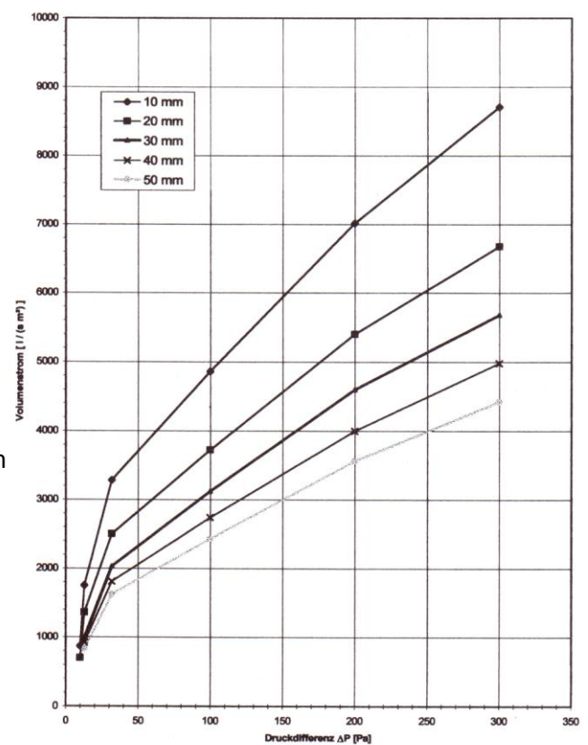
Luftwiderstandskurve PPI 20
