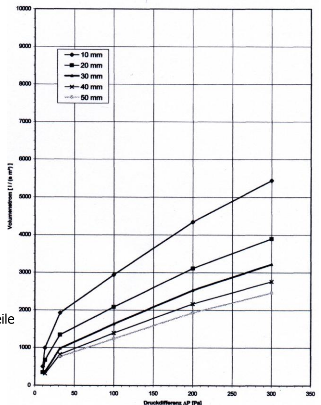
Luftwiderstandskurve PPI 45
